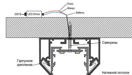
Светильник с выносным блоком питания
