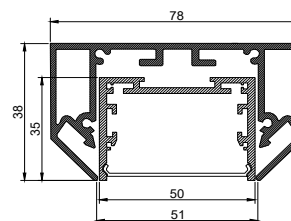
Светильник с выносным блоком питания
